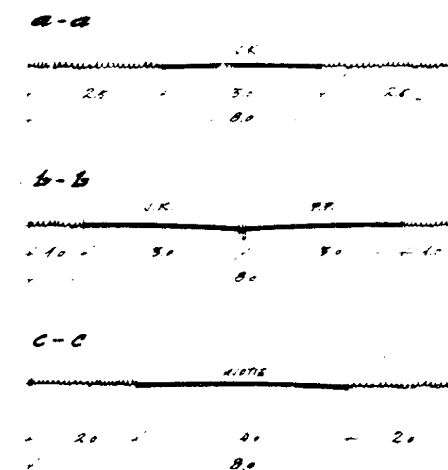
KATUJEN POIKKILEIKKAUKSIA 1:100
